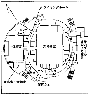
東総合スポーツセンターの平面図(上)と外観(左)
