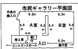
市民ギャラリー平面図
