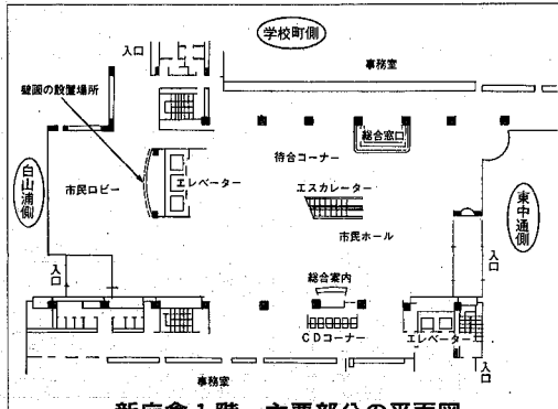
新庁舎1階・主要部分の平面図
