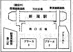
橋げた工事が完了した新潟駅西側連絡通路
