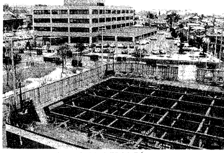
今年5月完成予定の雨水貯留池（西大畑町）
