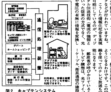
図2 キャブテンシステム
