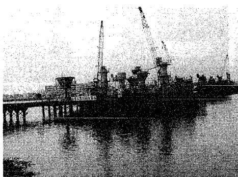
60年暫定2車線開通を目指し橋脚の建設工事が進む千歳大橋。新年度にはけた工事に着手します
