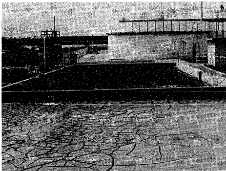
実験用に造った鳥屋野浄水場の天日乾燥床
