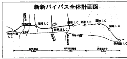
新新ハイパス全体計画図
