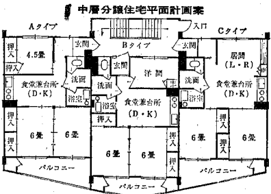
市民マンションの完成図
