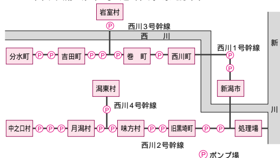
西川流域下水道幹線系統図
