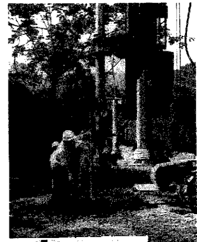
特殊改良工法としてのテノコラム工法の様子
