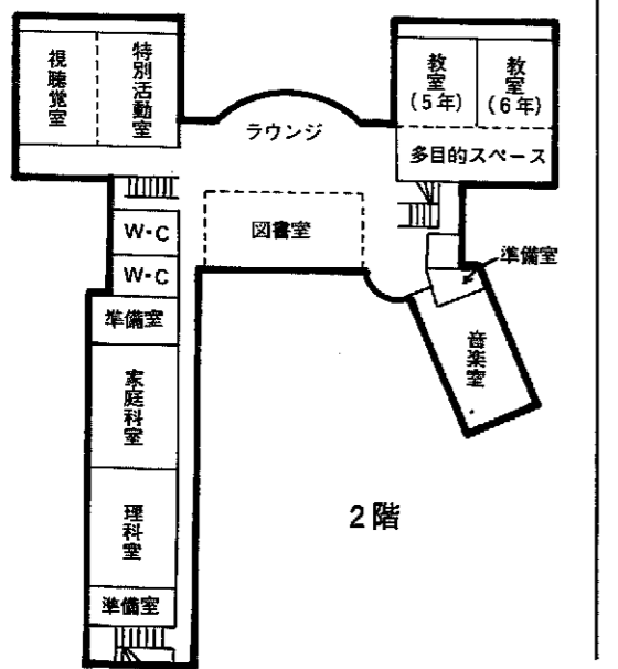
校舎平面図
