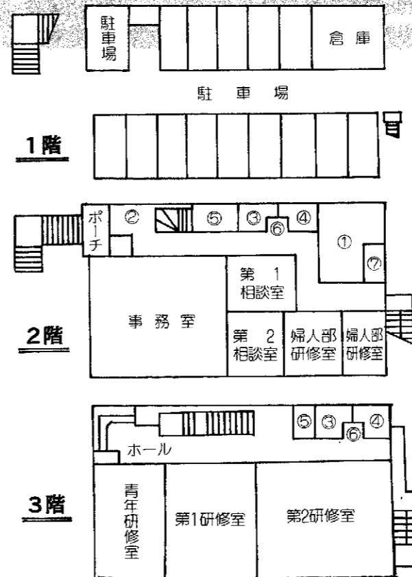
▲完成予想図
