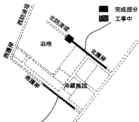
巻漁港計画図
