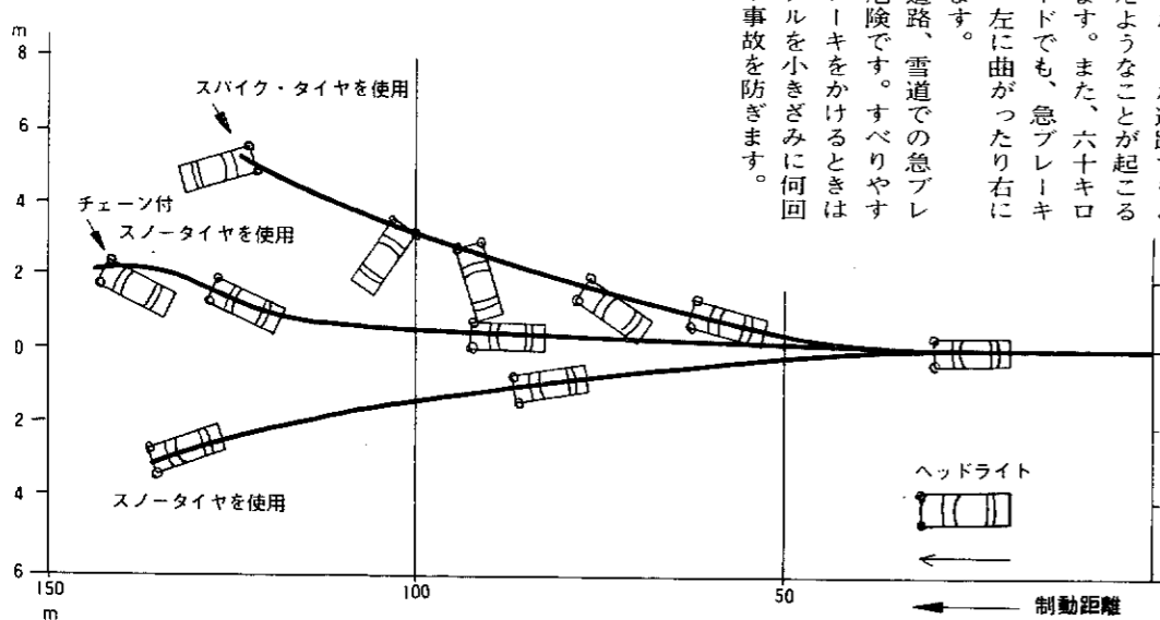
2000ccの乗用車が時速65.5km/hで直進中に急ブレーキをかけた場合(氷上)
