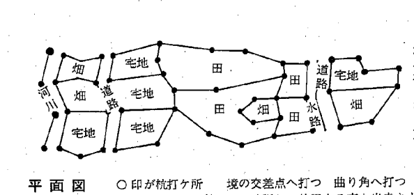
平面図 ○印が杭打ケ所 境の交差点へ打つ 曲り角へ打つ ○現在ある境界杭などは確認して使用する事も出来ます。
