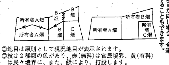
平面図 ○印が杭打ケ所 境の交差点へ打つ 曲り角へ打つ ○現在ある境界杭などは確認して使用する事も出来ます。
