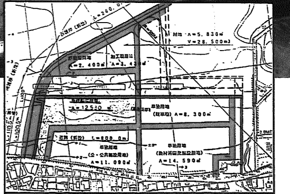
▲第1期漁港環境整備計画図
