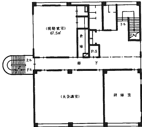
3階平面図
