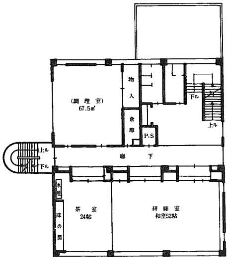
2階平面図
