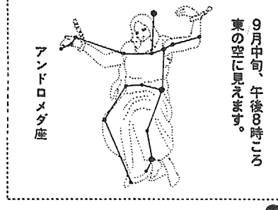
9月中旬、午後8時ごろ 東の空に見える。 ◆アンドロメダ座
