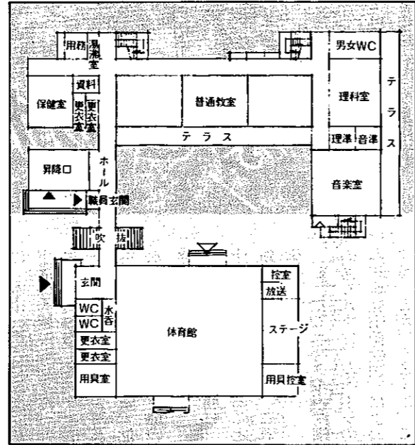
▲新飯田小1階平面図
