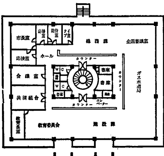
三階平面図
