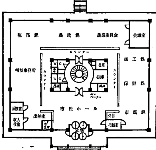
二階平面図
