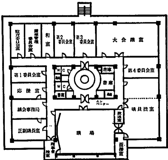
四階平面図
