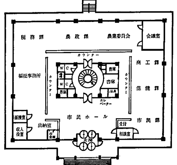
二階平面図
