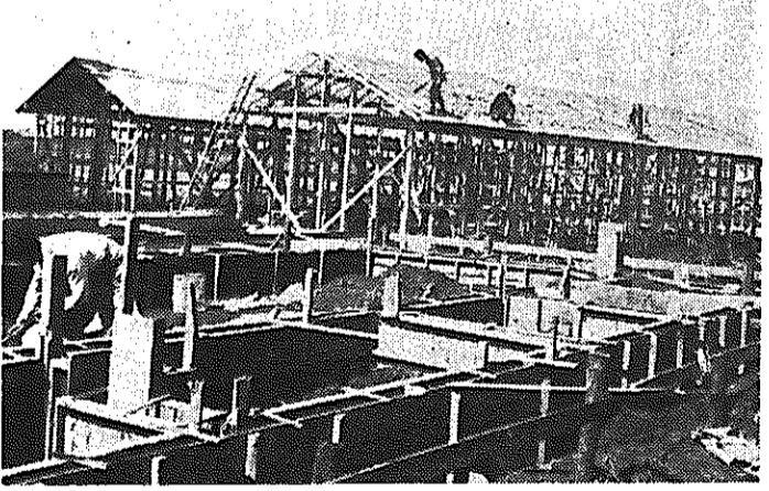
好天にめぐまれ仕事ははかどる工事現場
