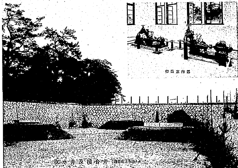
ポンプ室内部（右上写真）と取水井および接合井
