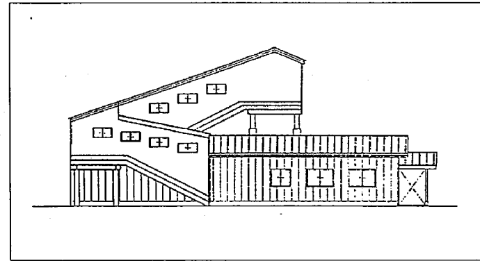
東側から見た亀田駅東口完成時の立面図
