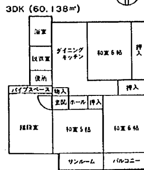
(平面図)
