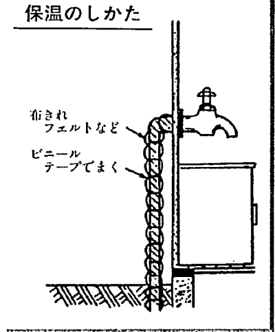
木枯らしの吹く季節になり、気温もだんだん下がってきました。とくに夜は寒さが厳しくなっています。本格的な雪が降る前に、水道管の冬じたくをして、凍結や破裂を防ぎましょう。
