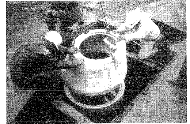
下水道マンホール布設状況
