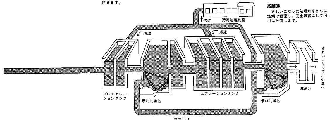
エアレーションタンク
