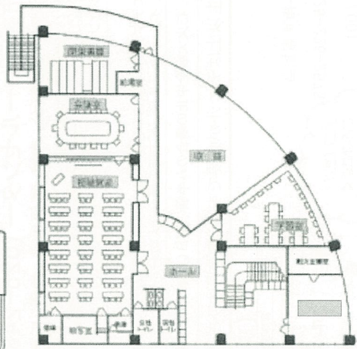
2階平面図
